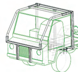
strutture di protezione a quattro montanti
