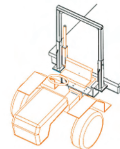
strutture di protezione a due montanti posteriori
